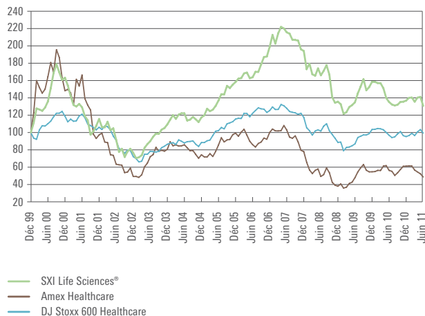
Graphique 4: Comparaison des performances de l'indice SXI Life Sciences®
